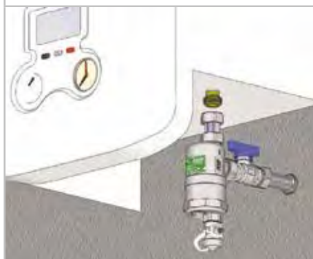
Пример установки грязеуловителя COMPACTFAR с телескопической муфтой (8882 1534)
